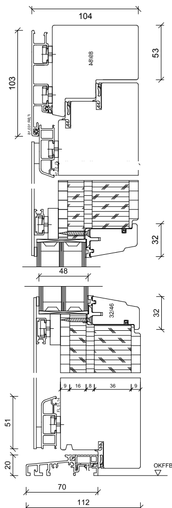
Abbildung: Schnitt AHT 3-105 Modern
