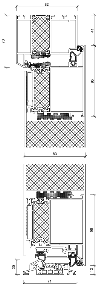
Abbildung: Schnitt und Musterecke AT 82 Design
