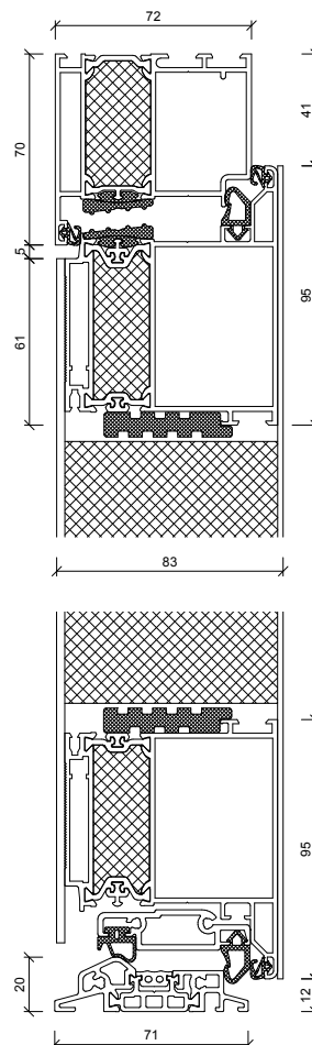
Abbildung: Schnitt und Musterecke AT 72 Exclusiv
