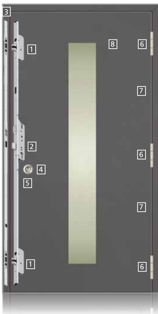
Abb.: Aluminium beidseitig flügelüberdeckend
